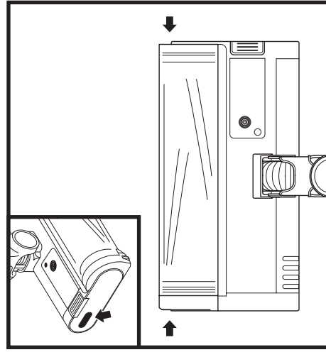
RENGJØRE EDGE DETECT-SENSOREN
