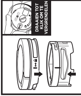
4. NIEUWE CARTRIDGE IN DRAAIKNOP PLAATSEN
