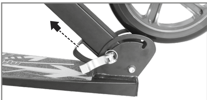
Kunststoffgriff nach oben ziehen, bis sich die Achse des Schnellverriegelungssystems aus der Halterung löst.
