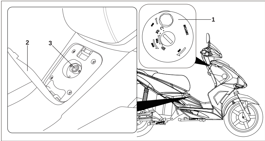
Abb. 4 Akku laden
