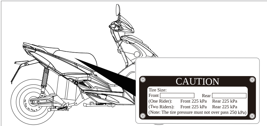
Abb. 11 Reifenluftdruck - Hinweisschild
