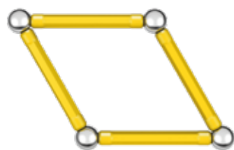
RHOMBUS
