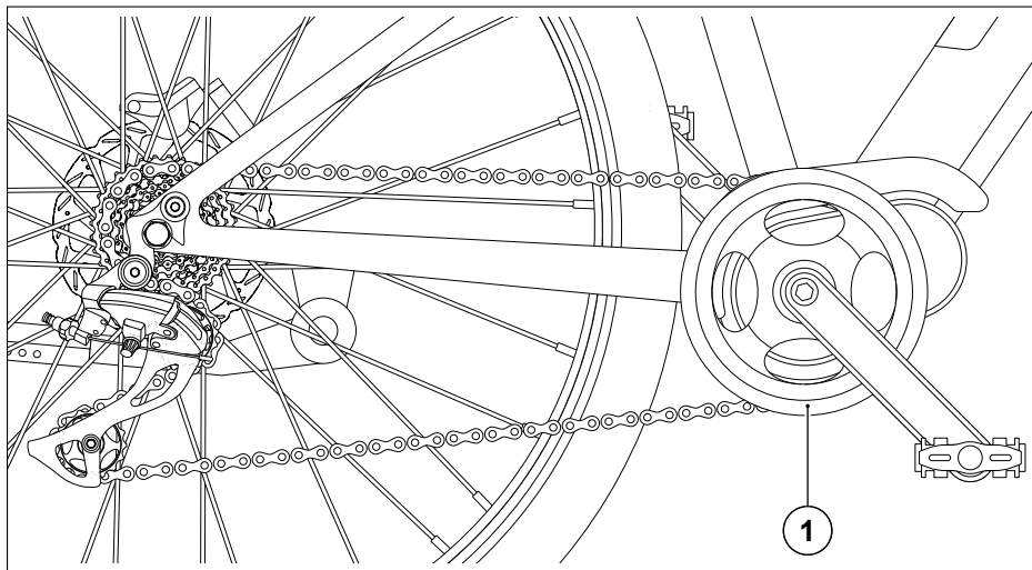
Abb. 24 Kettenschutz vorne
