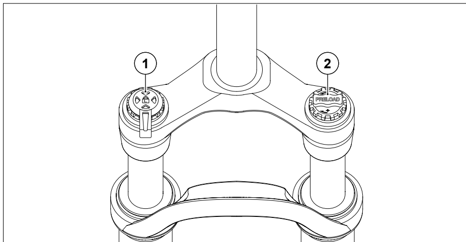
Abb. 18 Einstellbare Federgabel
