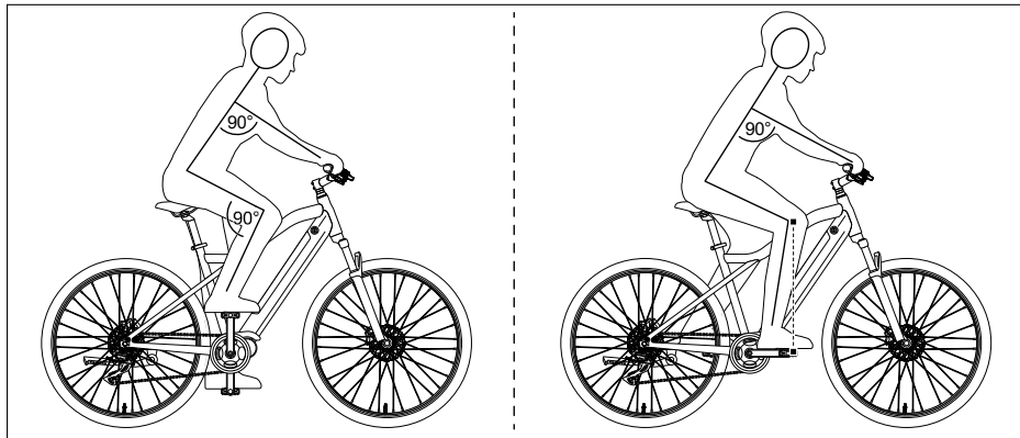
Abb. 4 Optimale Sitzposition
