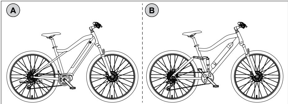
Abb. 19 Rahmentypen
