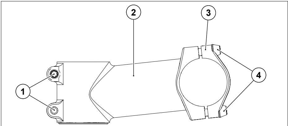
Abb. 34 Vorbau einstellen
