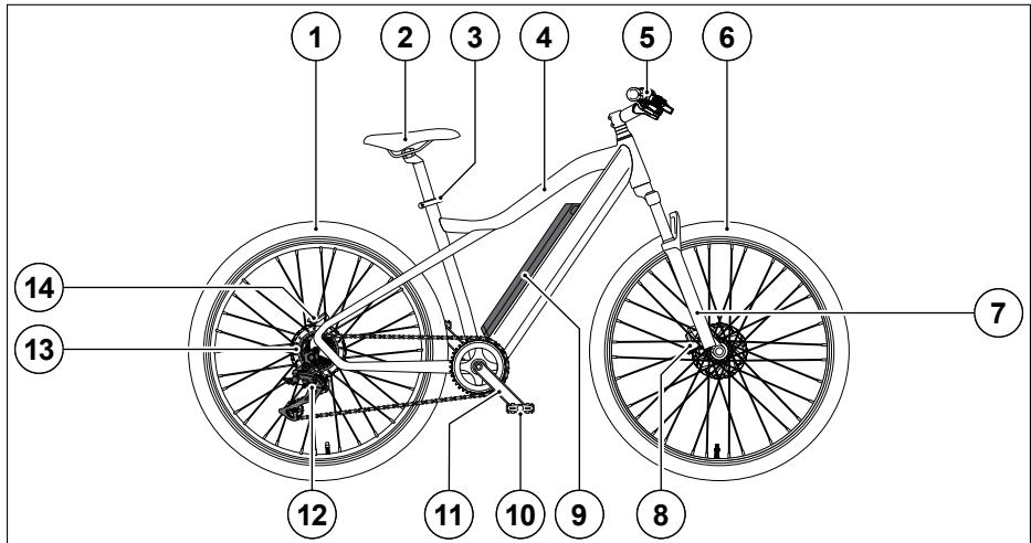
Abb. 6 Pedelec mit semiintegriertem Unterrohr-Akku, Hinterradmotor und Hardtail-Rahmen
