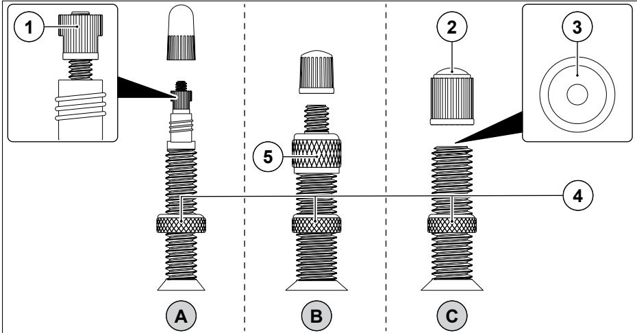
Abb. 30 Ventilvarianten
