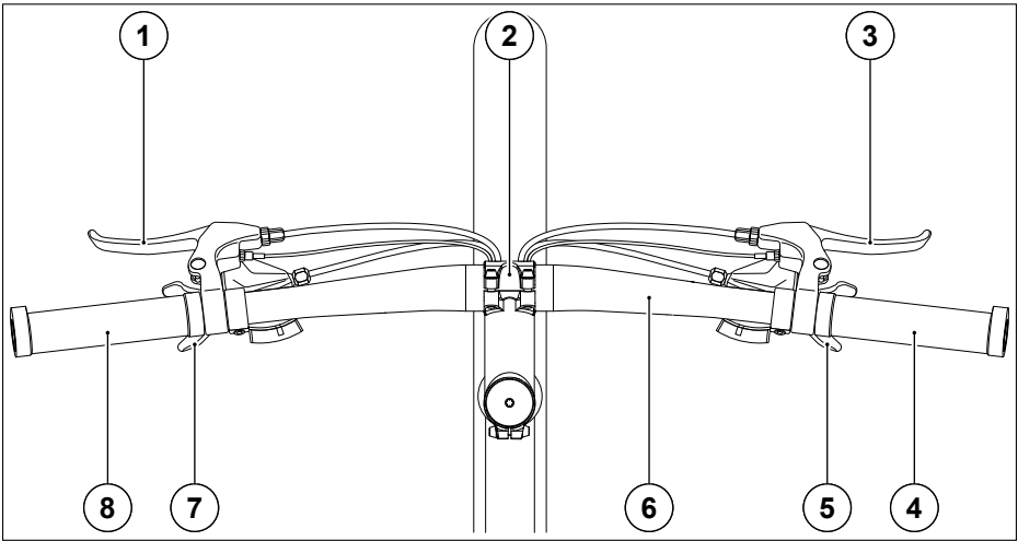
Abb. 33 Lenker und Vorbau
