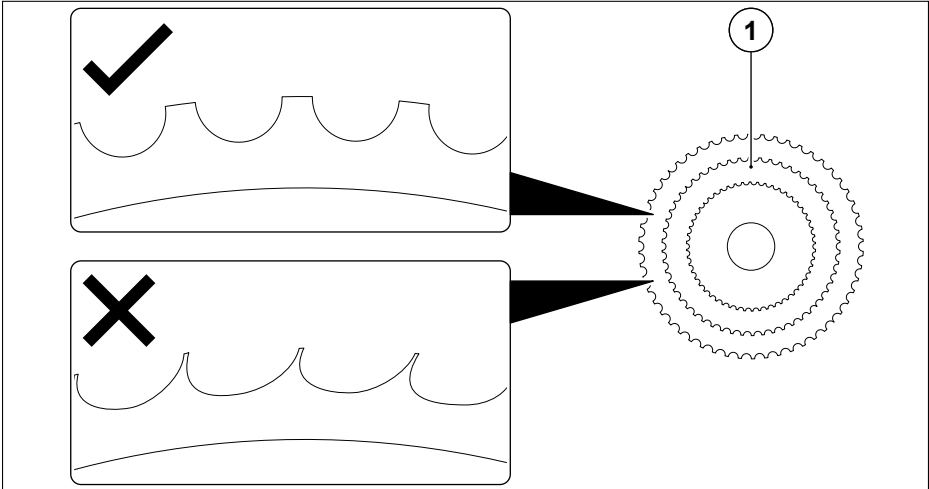
Abb. 37 Zahnkranzverschleiß
