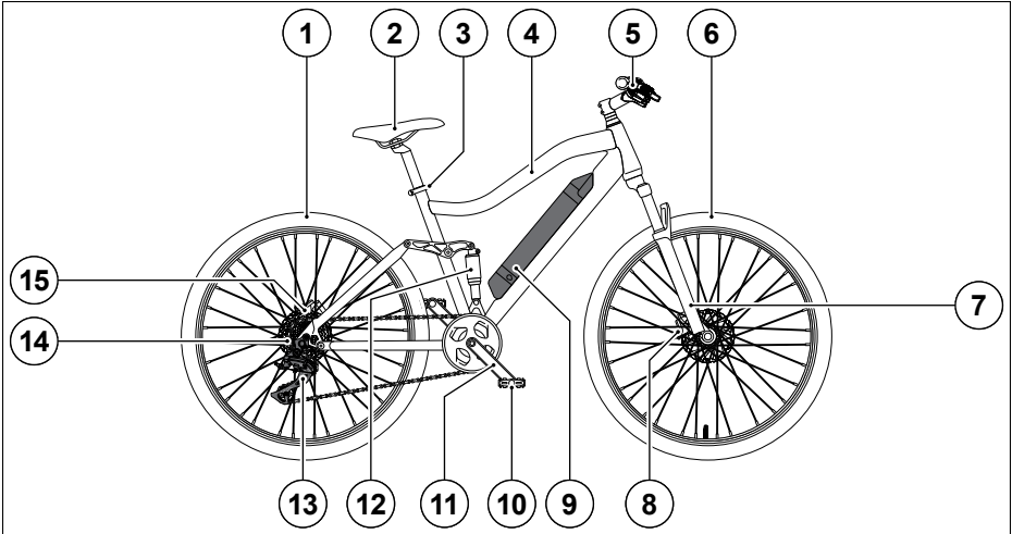
Abb. 7 Pedelec mit semiintegriertem Unterrohr-Akku, Hinterradmotor und Full-Suspension-Rahmen
