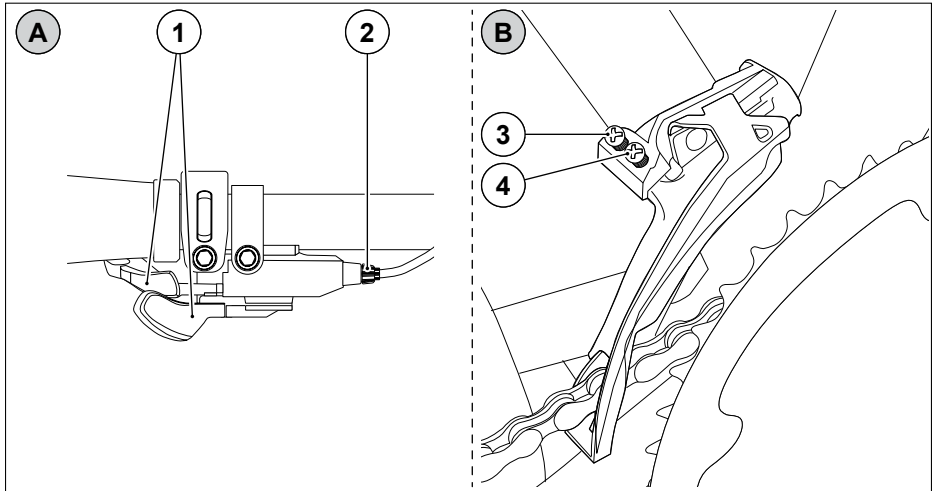
Abb. 39 Kettenschaltung vorne
