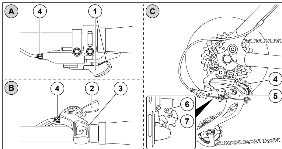
Abb. 40 Kettenschaltung hinten
