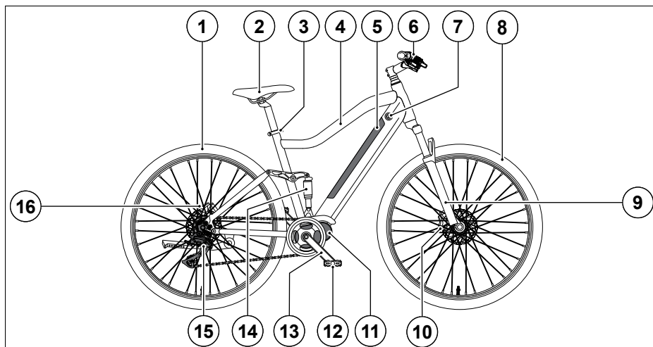
Abb. 10 Pedelec mit integriertem Unterrohr-Akku, Mittelmotor und Full-Suspension-Rahmen
