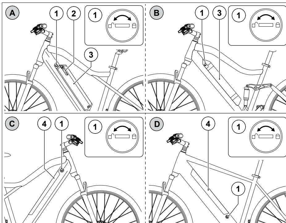
Abb. 11 Akku entnehmen/einsetzen
