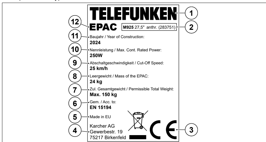
Abb. 1 Beispieltypenschild
