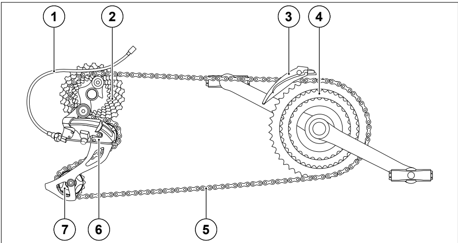
Abb. 22 Kettenschaltung
