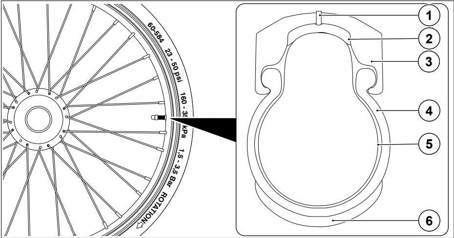
Abb. 29 Räder
