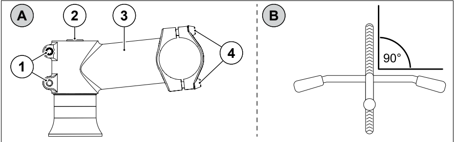
Abb. 35 Lenker einstellen
