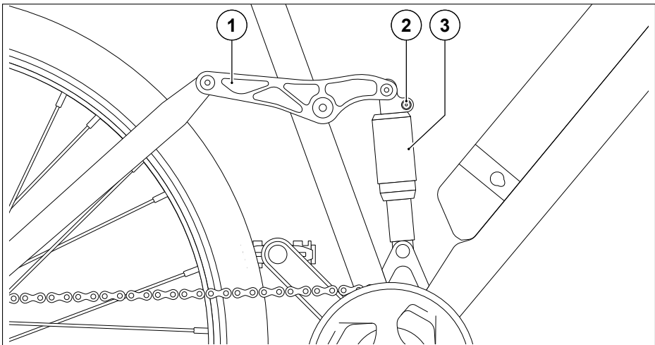
Abb. 20 Hinterbaufederung
