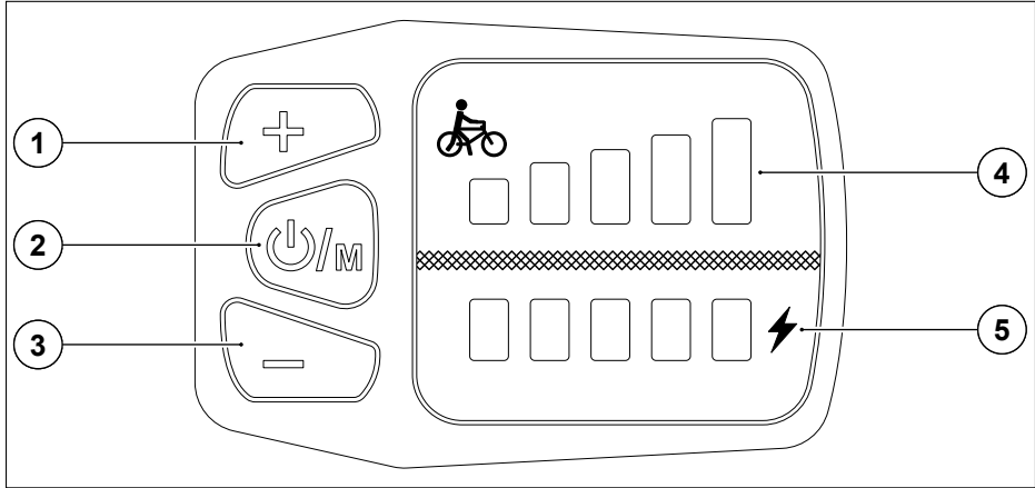
Abb. 16 Ananda D15
