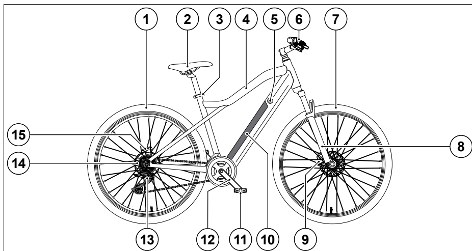
Abb. 8 Pedelec mit integriertem Unterrohr-Akku, Hinterradmotor und Hardtail-Rahmen
