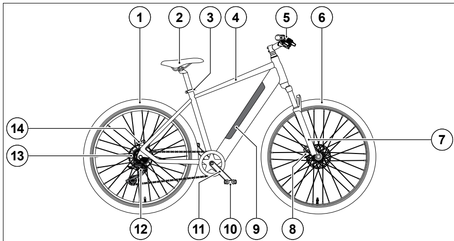
Abb. 9 Pedelec mit integriertem Unterrohr-Akku, Hinterradmotor und Hardtail-Rahmen
