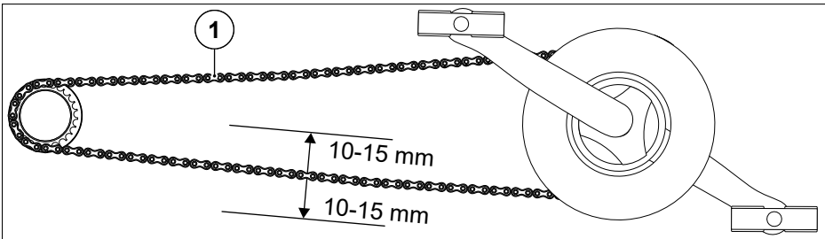
Abb. 38 Kettenspannung prüfen
