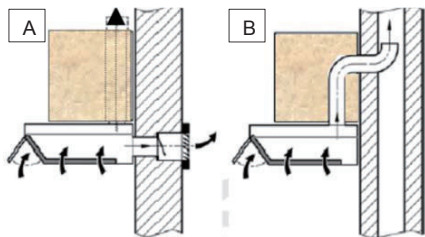
Fig. B Abluft über einen Luftschacht
