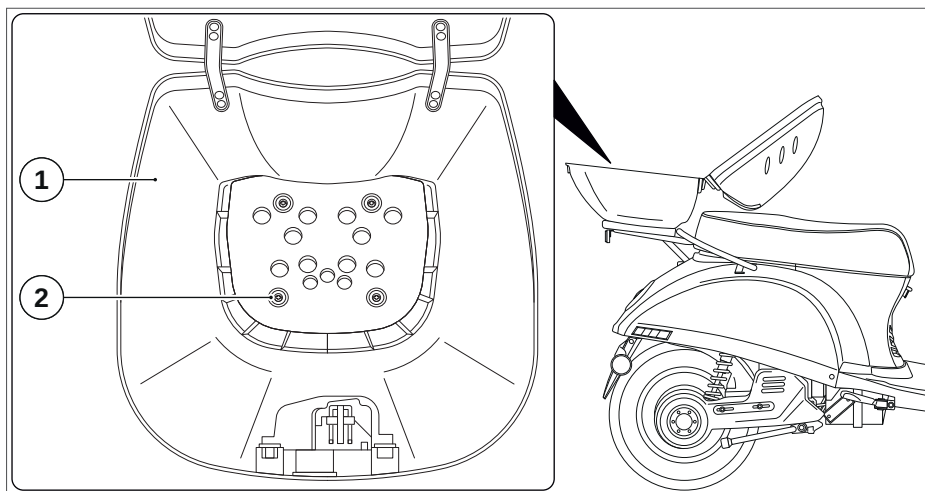
Abb. 10 Topcase montieren
