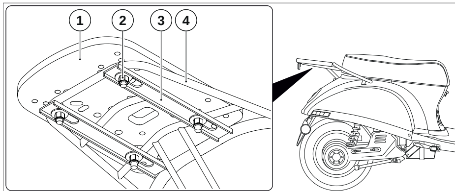
Abb. 9 Grundplatte montieren
