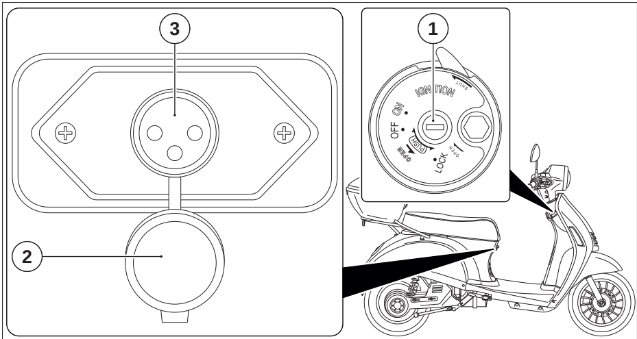
Abb. 4 Akku laden
