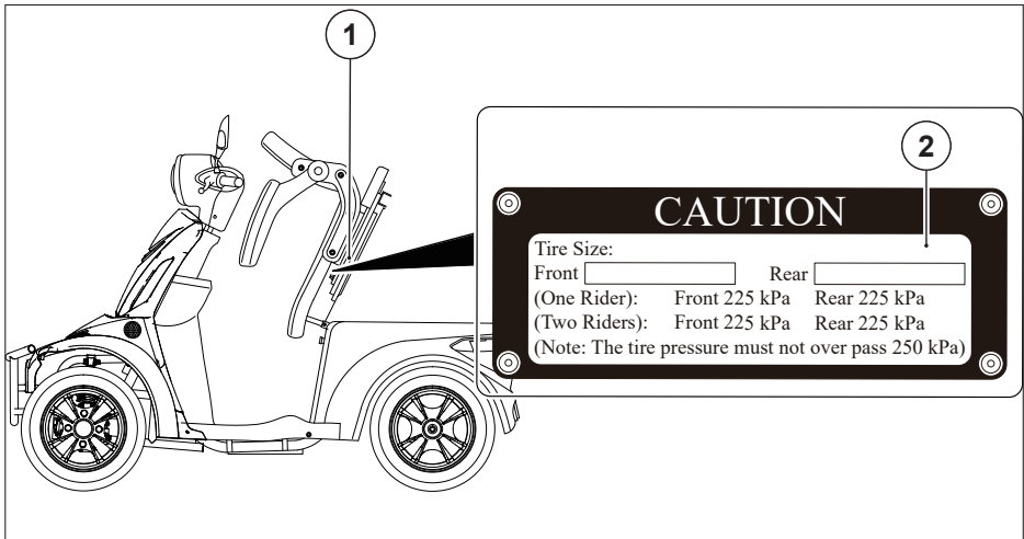
Abb. 15 Reifenluftdruck - Hinweisschild
