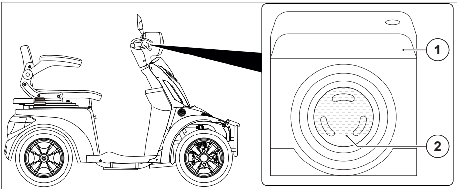
Abb. 13 Bremsflüssigkeit prüfen
