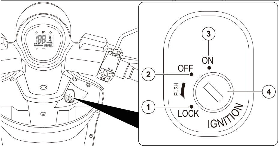
Abb. 8 Zündschloss (Beispieldarstellung)
