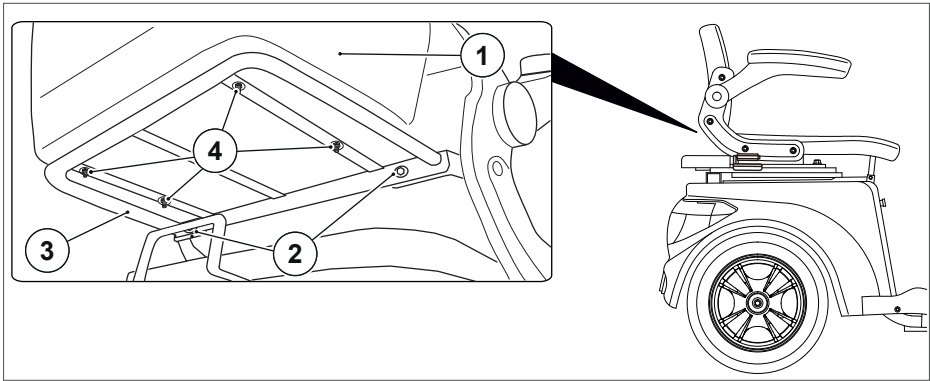
Abb. 11 Feststellbremse
