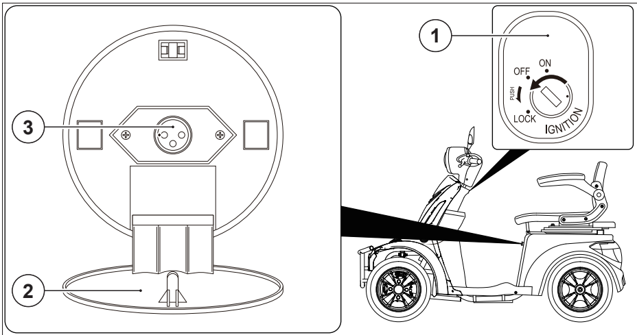
Abb. 5 Akku laden
