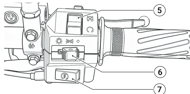
Abb. 10 | Bedieneinheit rechts
