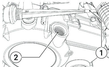
Abb. 22 | Ölstand prüfen
