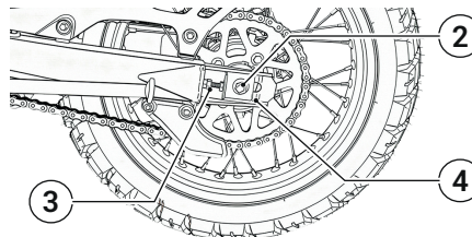
Abb. 37 | Kettenspanner
