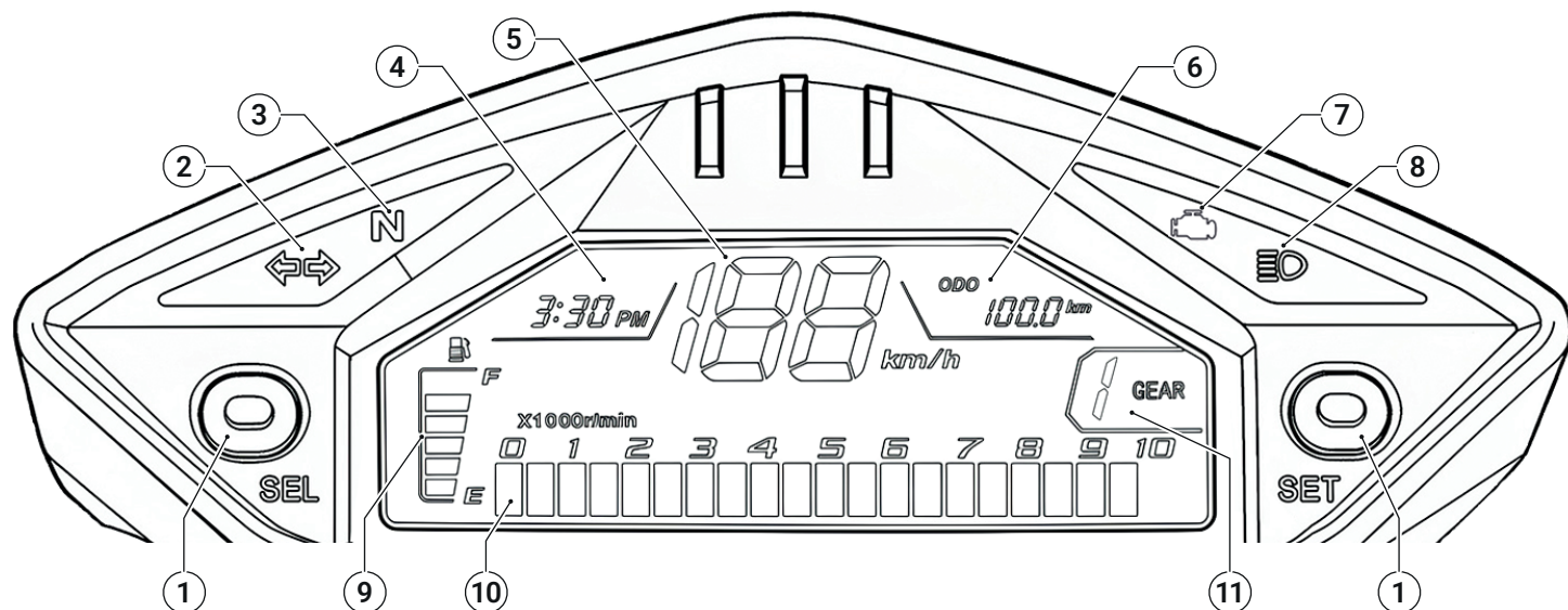
Abb. 5 | Instrumentenanzeige
