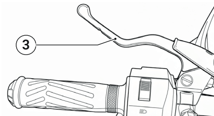
Abb. 15 | Bedieneinheit links
