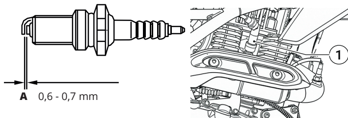
Abb. 20 | Zündkerze
