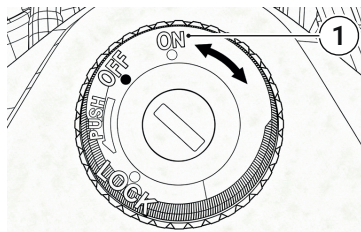
Abb. 13 | Zündschloss
