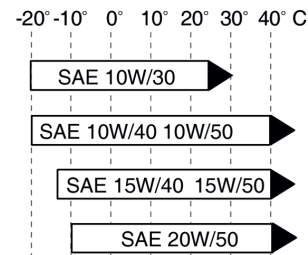
Abb. 24 | Empfohlene Viskosität in Abhängigkeit der zu erwartenden Außentemperaturen
