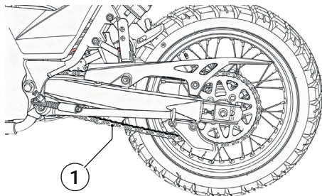
Abb. 36 | Antriebskette
