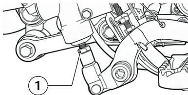
Abb. 32 | Einstellmutter Bremspedal-Spiel
