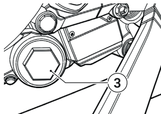
Abb. 23 | Ölablassschraube
