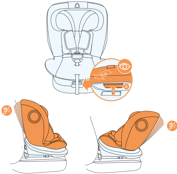
A: Hebel zur Einstellung der Rückenlehnenneigung
