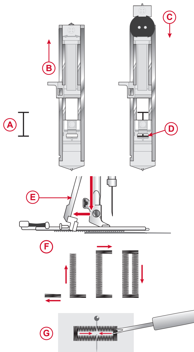
Einstellung für Knopfloch
