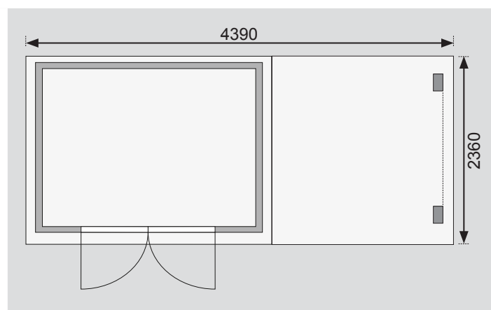
Draufsicht (in mm)
