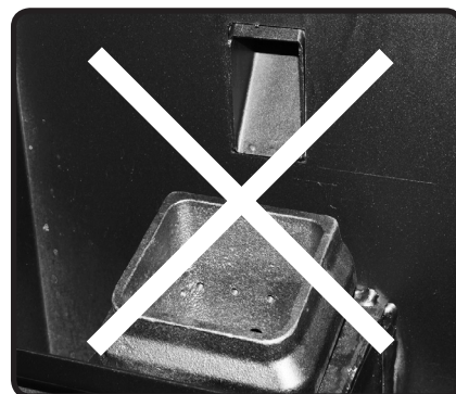
Abb. 8c: Falsch eingesetzter Brenntopf
