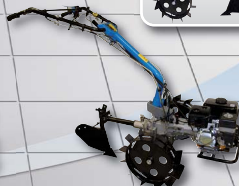
Abb. Pflug montiert an Motoreinachser
