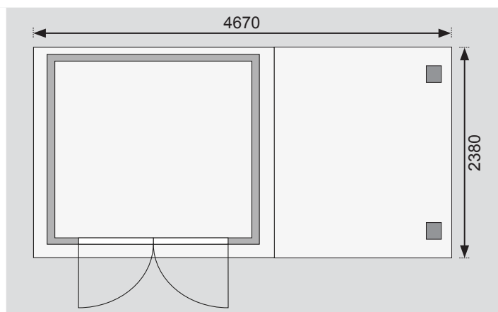
Draufsicht
