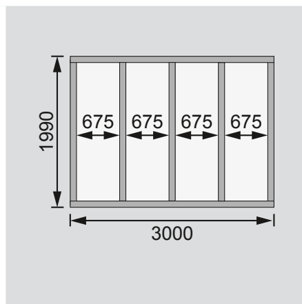
Fundamentplan mit Boden (in mm)
