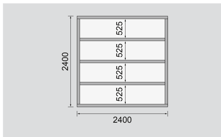
Fundamentplan mit Boden (in mm)
